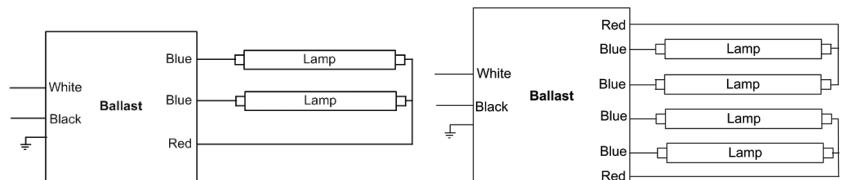
(1) 2-lamp wiring
